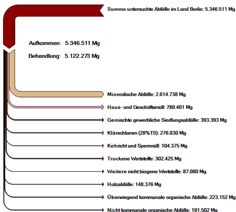
Abbildung 2.4: Sankeydiagramm Mengenströme 2022
